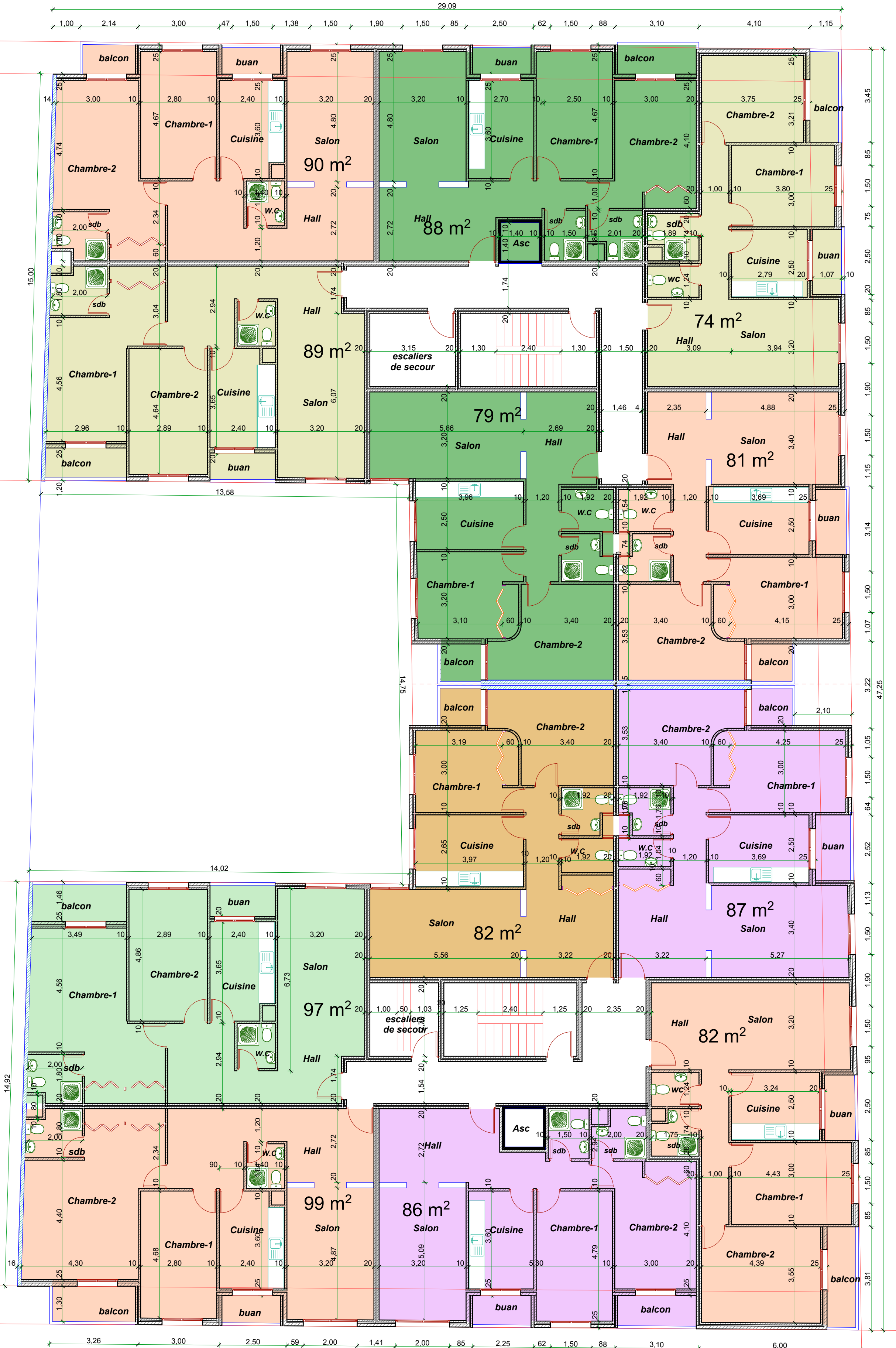
Etage courant
